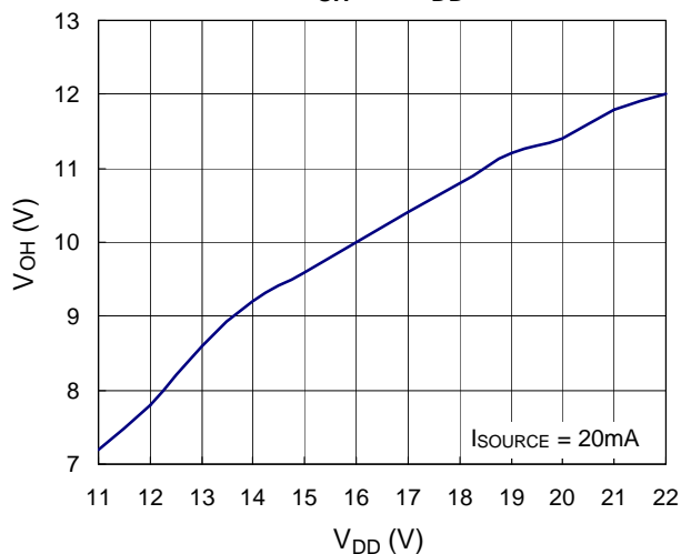
V_{OH} vs. V_{DD}
