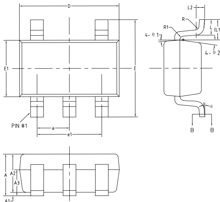
SOT23-5
