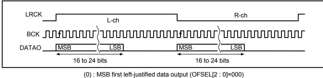
(0) : MSB first left-justified data output (OFSEL[2 : 0]=000)
