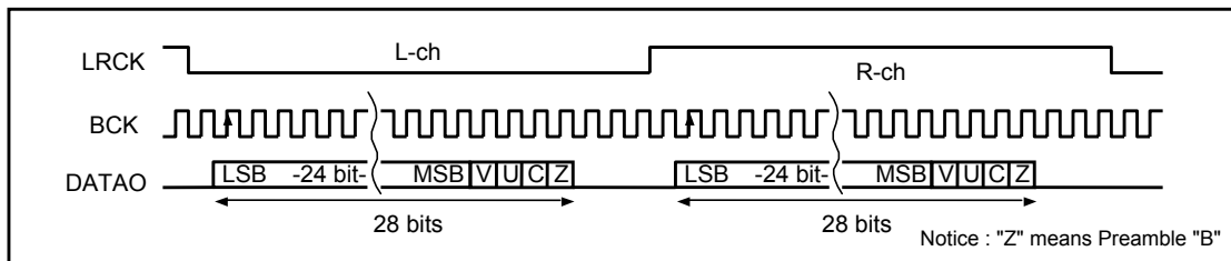
(4) : NRZ data I 2 S output (OFSEL[2 : 0]=110)
